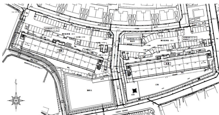
配置図
